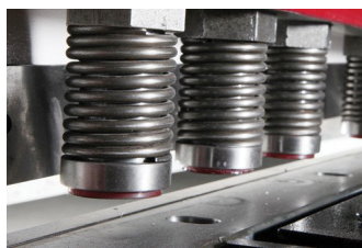
Blechniederhaltersystem
